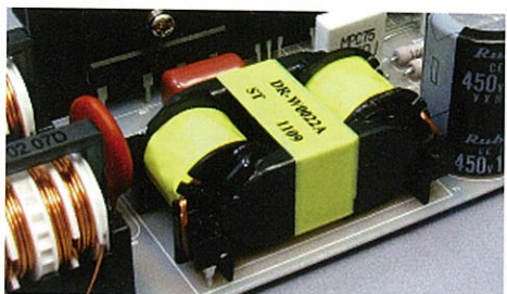
リンクトランスコア(実装写真)
