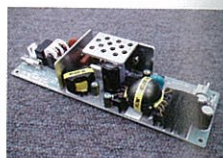
LED照明用電源
